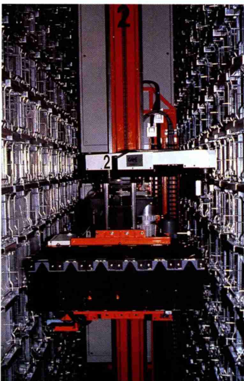
20 Robot serveur de livres (trans-stocker «GAME») dans les magasins de la bibliothèque municipale de Bordeaux
