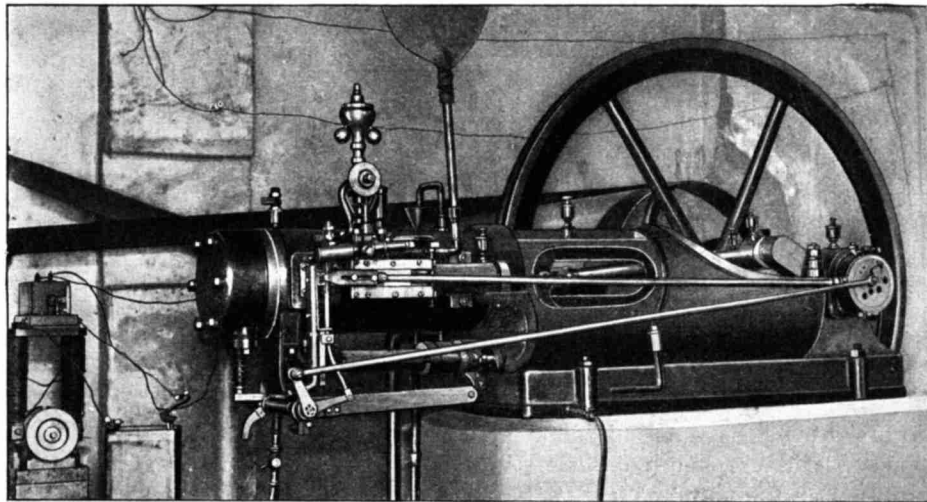
Fig. 13. Seitenansicht der 4pferd. Gasmaschine.
