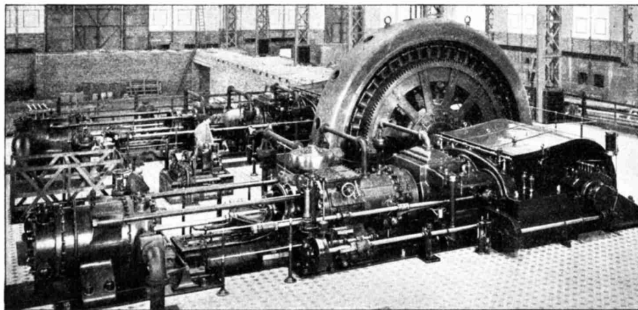
Fig. 26. 1000pferd. Gasdynamo der Kraftzentrale der Ilseder Hütte. (Oechelhaeuser-Maschine der Walchener Maschinen-A.-G.)
