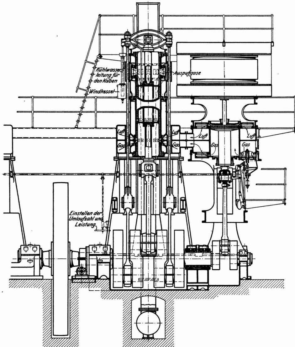
Fig. 34. Stehende Oechelhaeuser-Maschine mit Gebläse gekuppelt. Zwillingsanordnung.
