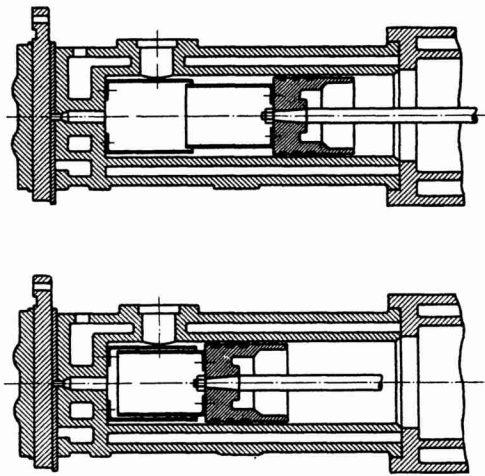
Fig. 1. Vorversuche an der Ottoschen Gasmaschine im Jahre 1886.
