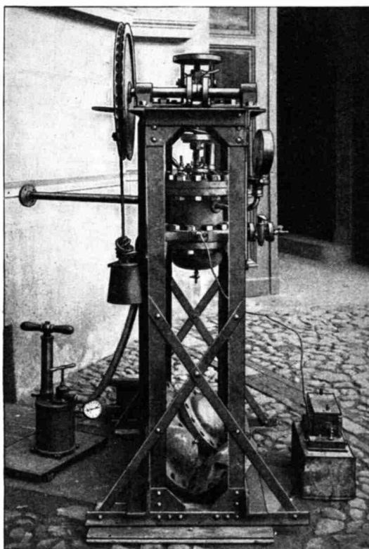
Fig. 3. Oechelhaeusers Apparat für Verbrennungsversuche von Gasen 1886 bis 1887.
