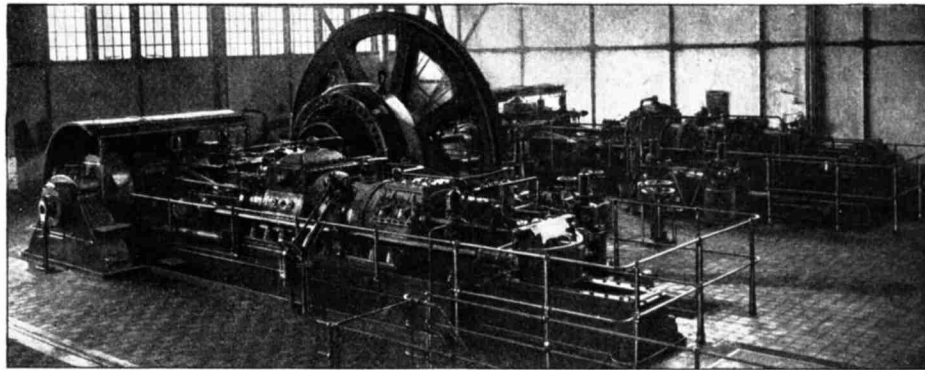
Fig. 27. 1000pferd. Oechelhaeuser-Maschine der Alpinen Montan-Gesellschaft in Donawitz (Steiermark).
