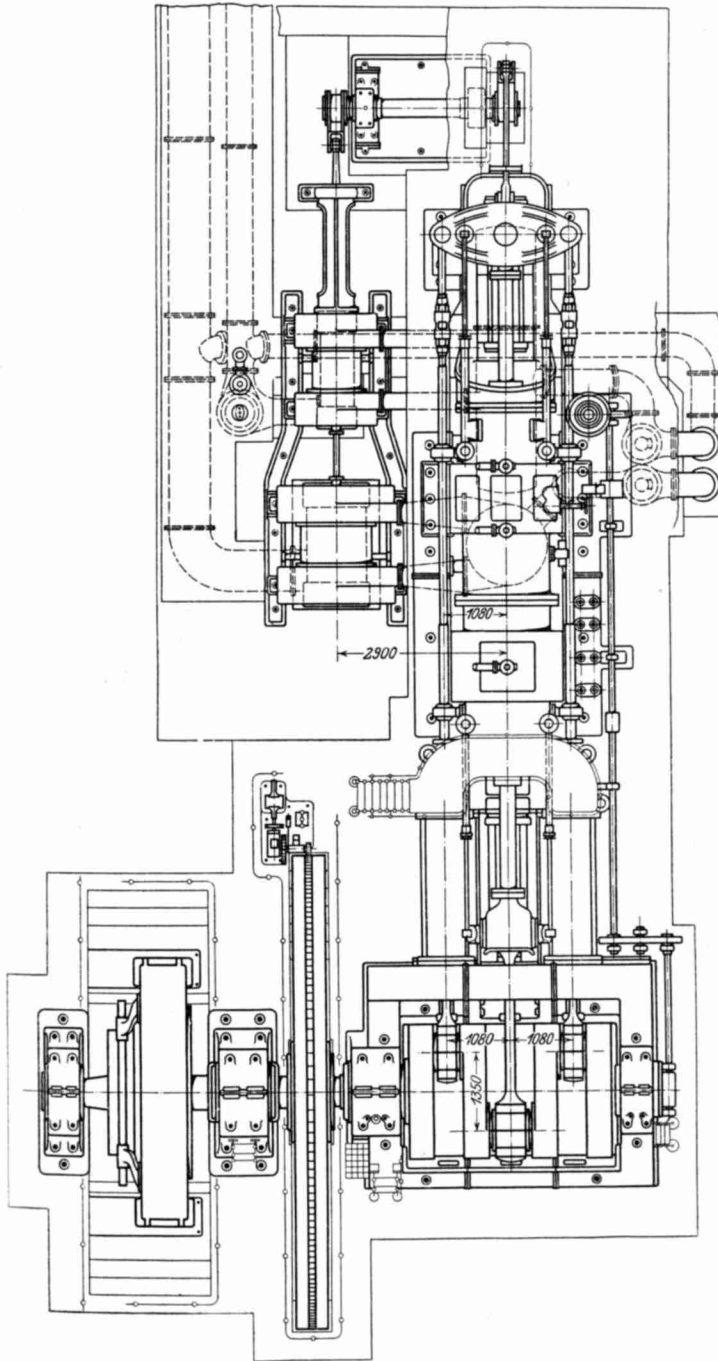
Fig. 28 bis 30. Großgasmaschine von 1800 PS., System Oechelhaeuser. (Erbaut von A. Borsig.)
