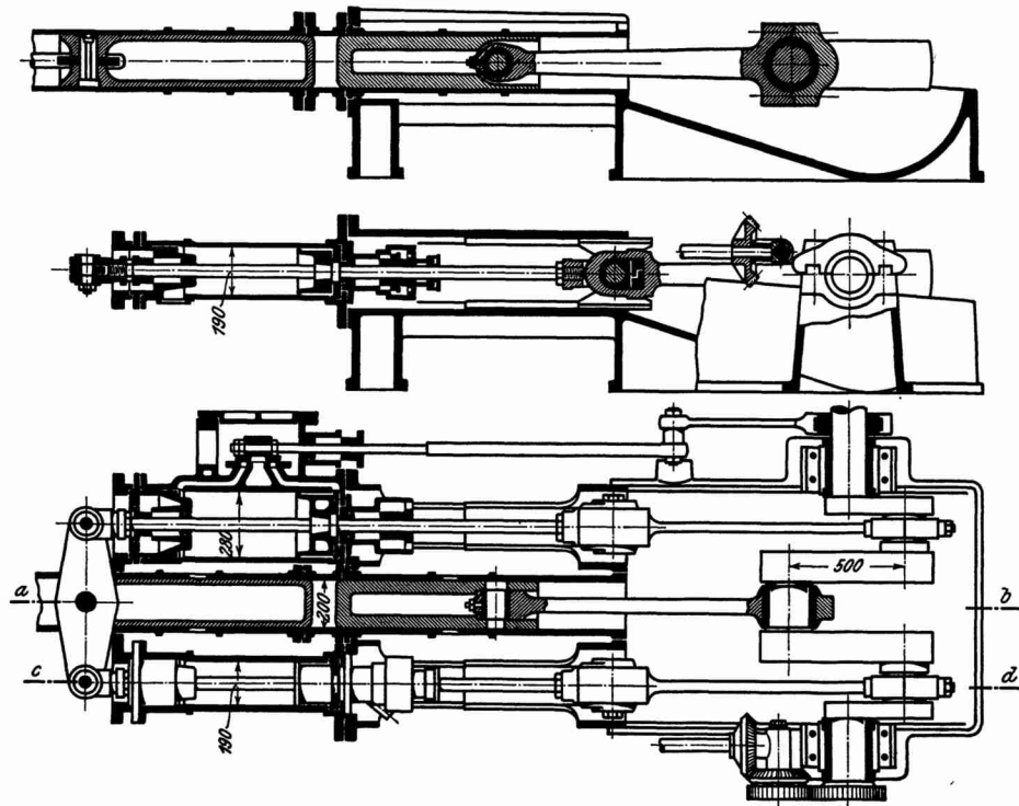
Fig. 14 bis 16. Doppelkolbenmaschine 1892.
