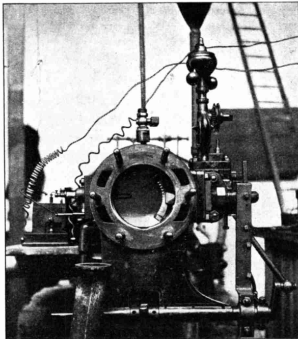
Fig. 21. 4 pferd. Benz-Gasmaschine 1887.
