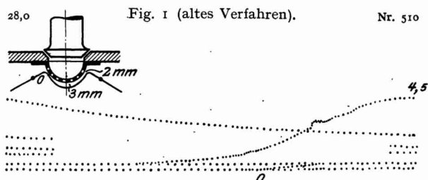
Späte Zündung, starkes Nachbrennen. Ohne Ventil. Gasmenge = 460 \div 620 ccm. Gas : Luft = 1 : 3,6 \div 2,6.
