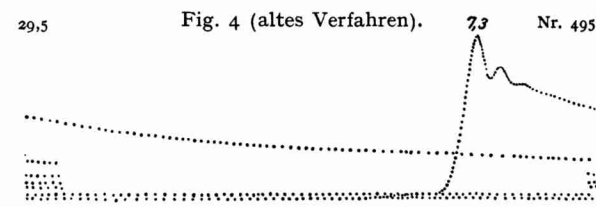
Verspätete Zündung, hoher Verbrennungsdruck. Ohne Ventil. Gasmenge = 250 \div 260 ccm. Gas : Luft = 1 : 6,6 \div 6,3.
