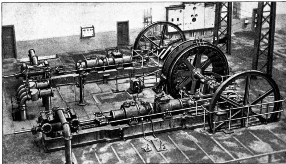
Fig. 23. 600pferd. Gasdynamo (erste Großgasmaschine), in Betrieb gesetzt am 12. Mai 1898 im Hörder Bergwerks- und Hüttenverein.
