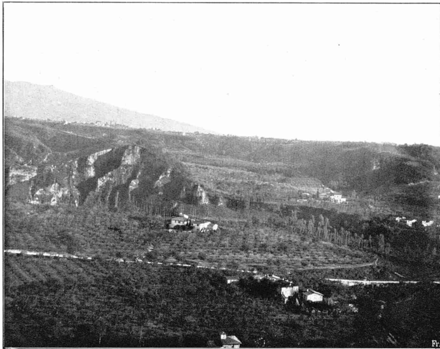
Abbild. 45. Tal des Torrente Resco, das einen Schwemmkegel am Fuße des Monte Pratomagnogebirges durchschneidet (nach Südosten gesehen).
