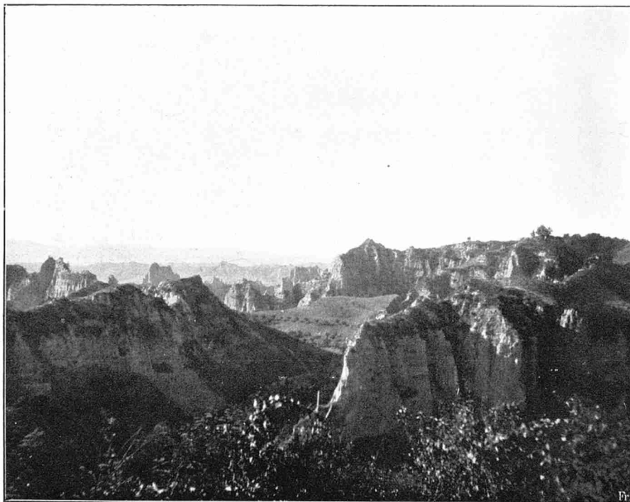
Abbild. 46. Badlands nahe dem Torrente Resco, gegenüber Figline.
