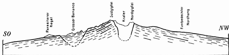
Abbild. 65. Profil durch den Rofs-Berg in den natürlichen Böschungsverhältnissen.
