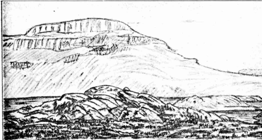
Abbild. 64. Rundhöcker mit Stofs- (rechts) und Leeseite (links). E. Werth gez.
