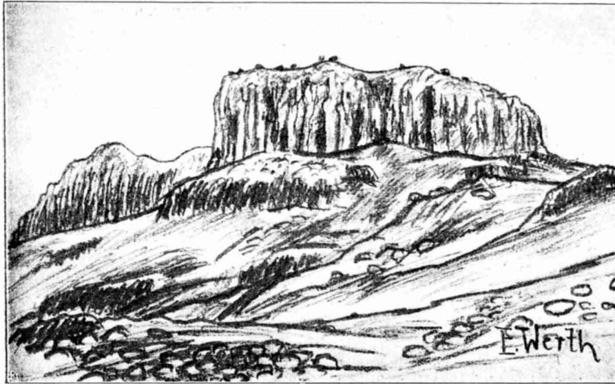
Abbild. 63. Steilwandiger Basaltklotz.
