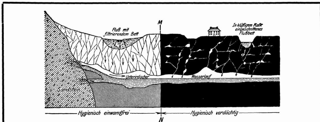
Abb. 192. Hygienisch verschiedenes Verhalten der Strecken eines unterirdischen Wasserlaufs
