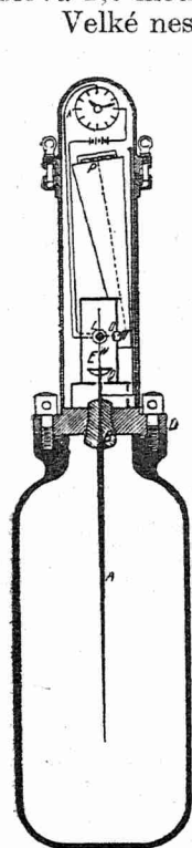
Obr. 1. Regenerova „regi- strační bomba“. Je vodotěsná a obsahuje vedle ionisační komory jednovláknový elektrometr a re- gistrační zařízení s hodinovým strojem.
