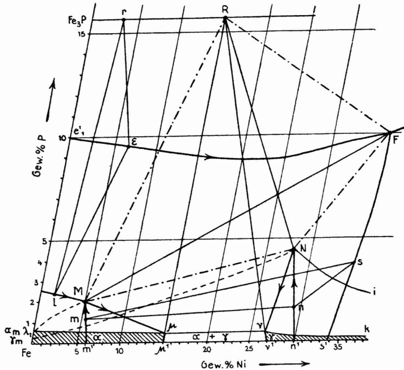
Fig. 2. Die Eisenecke des ternären Zustandsdiagramms Fe-Ni-P nebst Isothermen bei 400^{\circ} .
