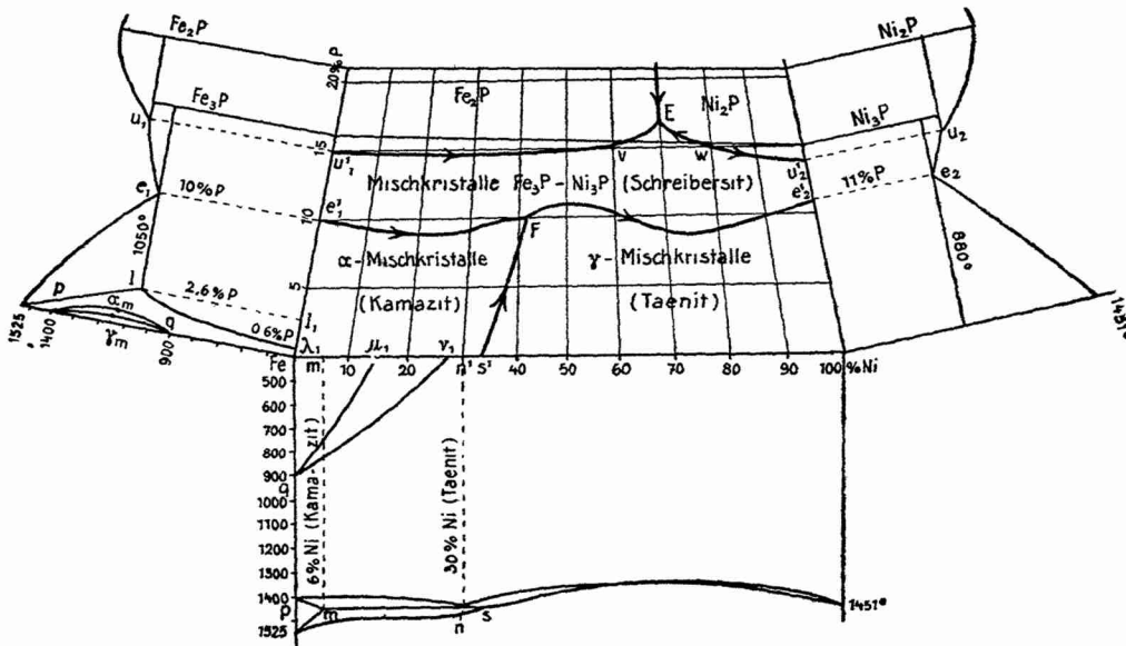
Fig. 1. Übersicht über das ternäre System Fe-Ni-P.
