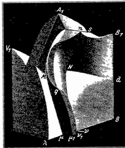
Fig. 3. Modell des ternären Zustandsdiagrammes Fe-Ni-P.
