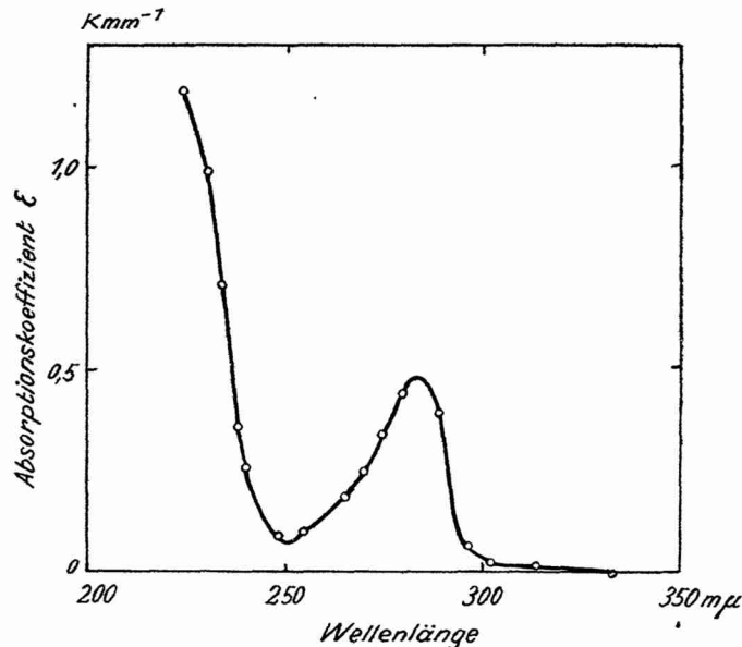
Fig. 1. Absorptionsspektrum einer 0,027% cgm alkoholischen Hormonlösung.
